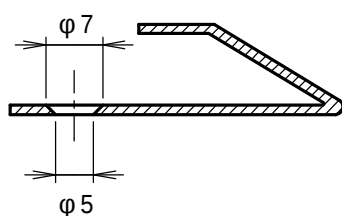
S1-S1断面図 (1/1)
